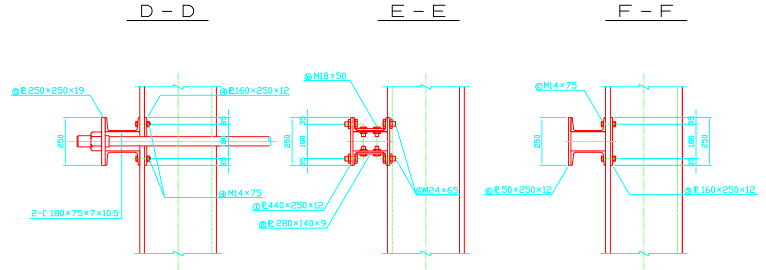
プレート詳細図 s=1:5
