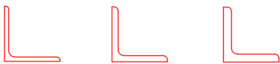
L-90x90x7 L-90x90x10 L-90x90x13
