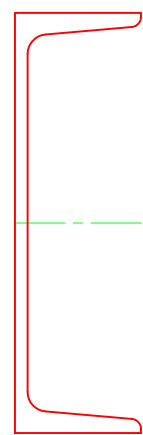
C-300x90x9x13
