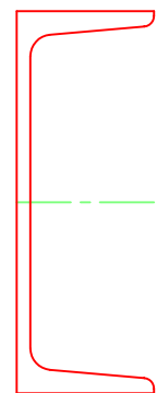
C-250x90x9x13
