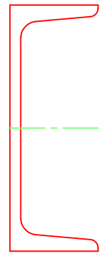
C-250x90x11x14.5
