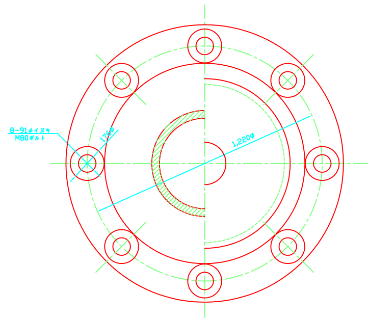
断面 A-A
